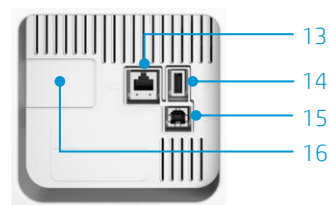
Vista ampliada del panel de E/S posterior
